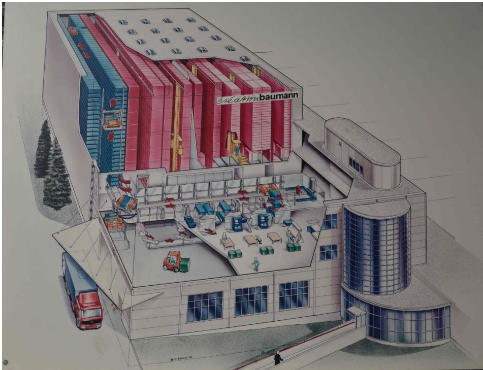
Systematisch dargestelltes Materiallager (Hochregallager)
